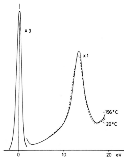
Abb. 1. Energieverlustspektren für eine 850 Å dicke Bleischicht mit 50 kV-Elektronen in einem Streuwinkel \vartheta = 2 \cdot 10^{-2} rad. Die beiden Kurven wurden bei \Delta E = 0 aneinander angepaßt.
